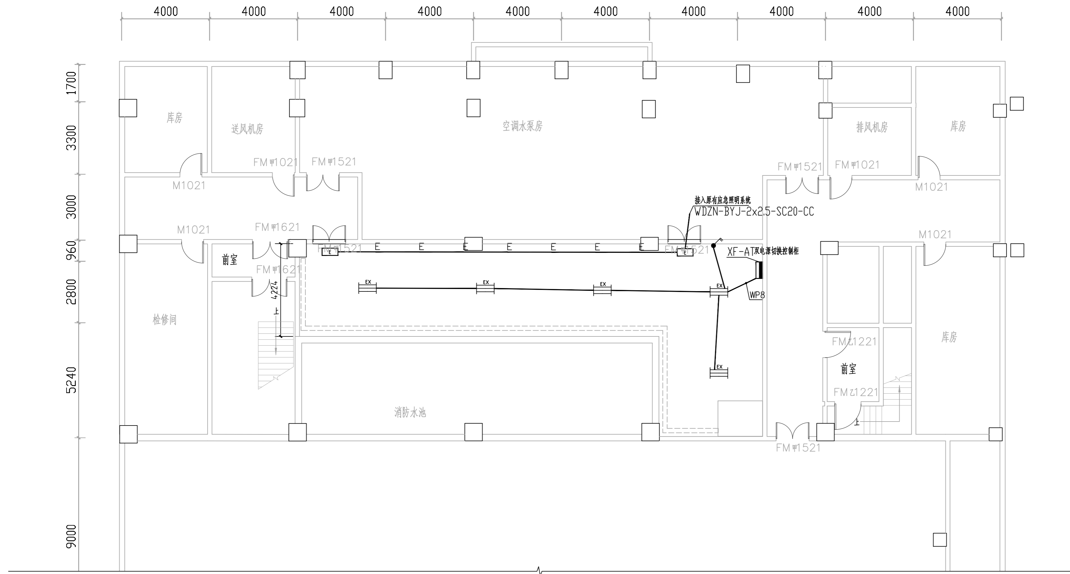
水泵房备用照明布置图 1:100
